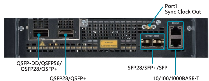
400G (QSFP-DD) Multirate Module MU104014B
