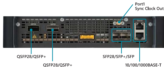
100G Multirate Module MU104011A
